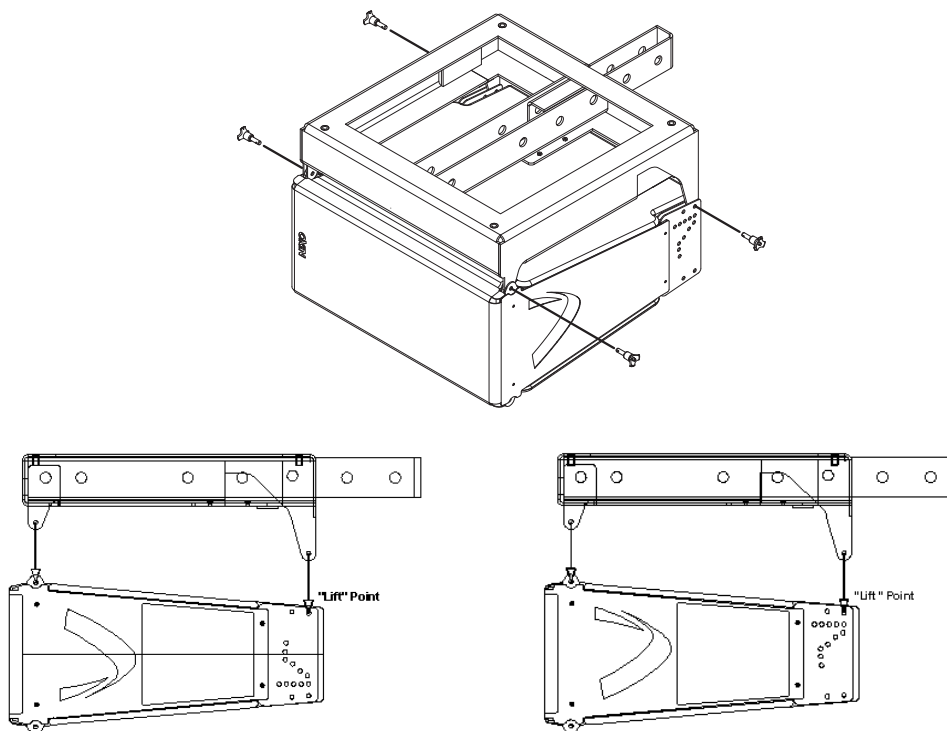
最初の GEO D10 とバンパーの結合
