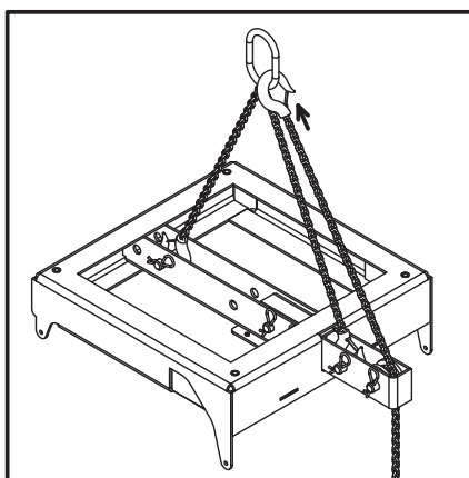
モーター、ブライドル、ホイール、およびチェーンレベルホイス্টの接続
