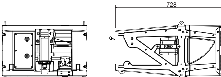
背面図
