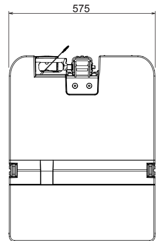
上面図
