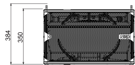
正面図
