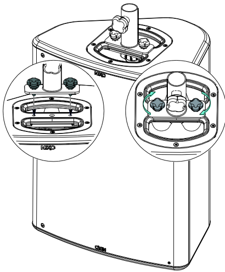
Avec l'enceinte
