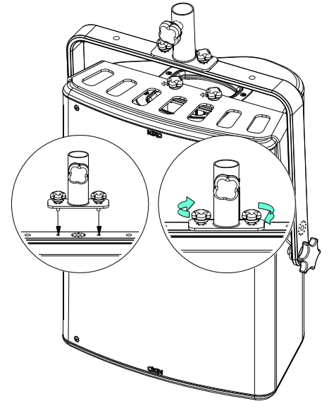
Avec VBRK
