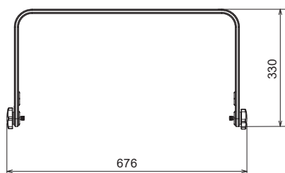
正面図
