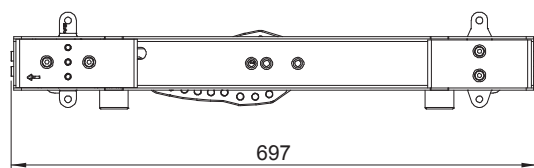
左側面図
