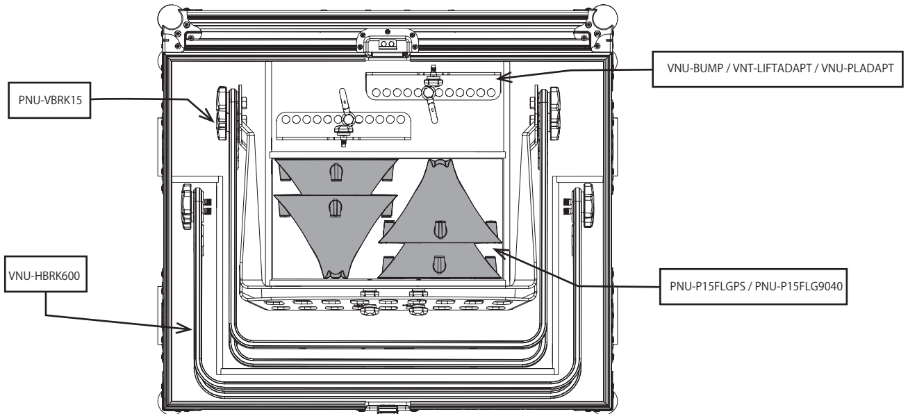
正面図
