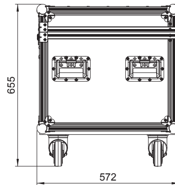
右側面図
