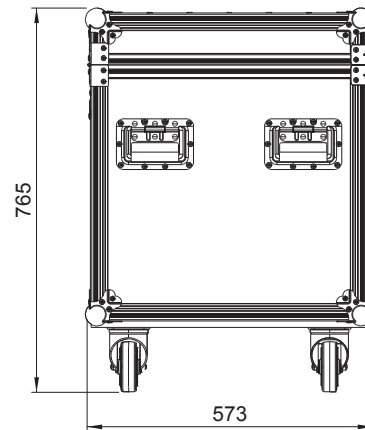
右側面図
