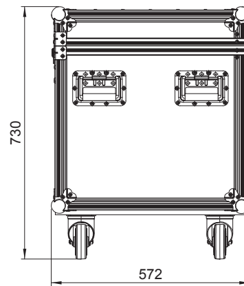
右側面図
