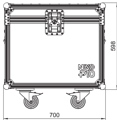
正面図
