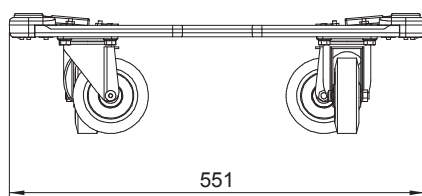
正面図
