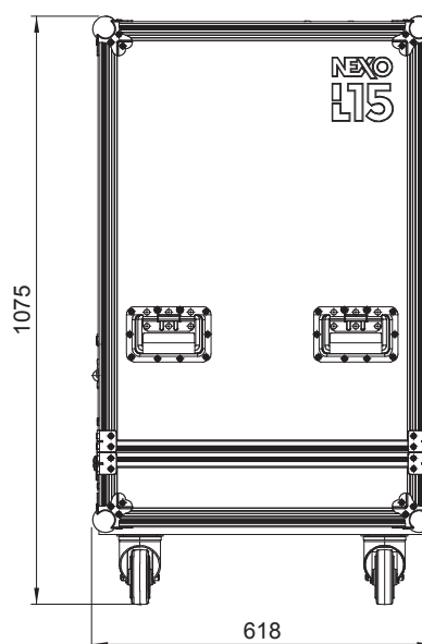
右側面図
