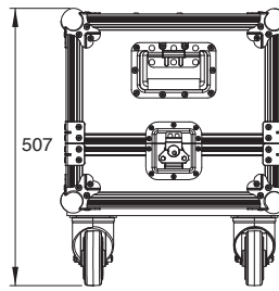
右側面図
