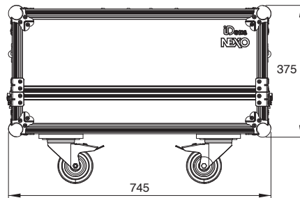
正面図
