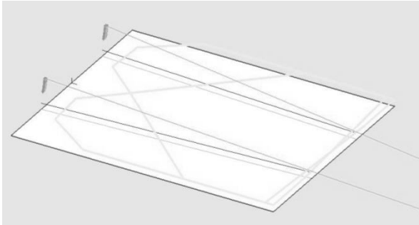
Couverture à -6 dB, avec toutes les enceintes GEO M10 en configuration 80°
