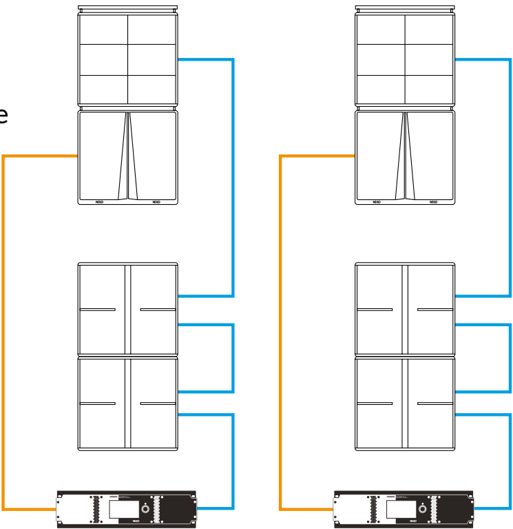
1 B218 + 1 M210 + 2 L20 amplifiés par 1 NXAMP4X4MK2 par côté
