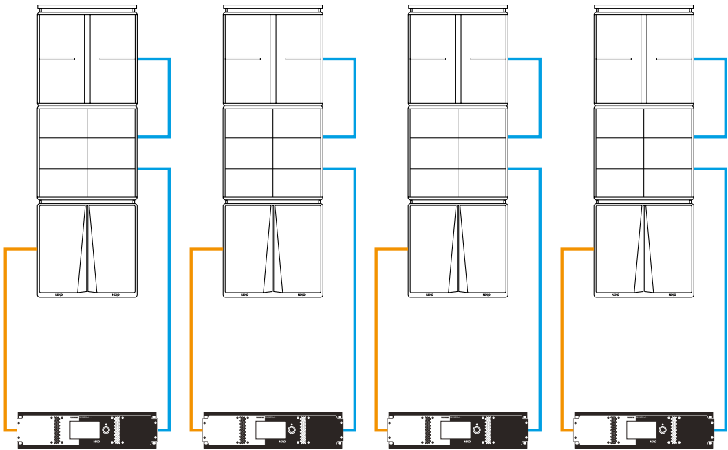
1 L20 + 1 B218 + 1 M210 amplifiés par 1 NXAMP4X4MK2 par cluster
