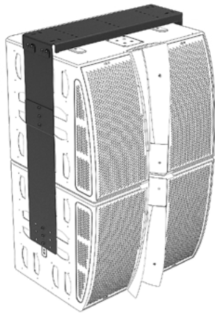
ANI-LK01 M210 sous M210
