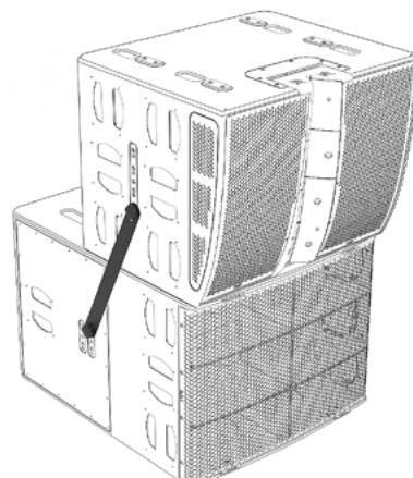
VNT-CPL04 Lien L20 / B218 / M210
