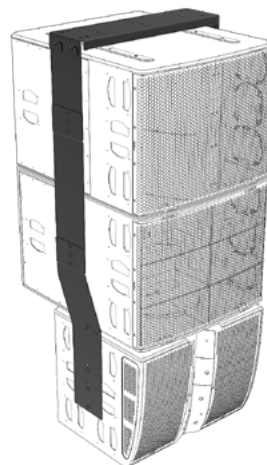
ANI-LK03 M210 sous B218 et L20
