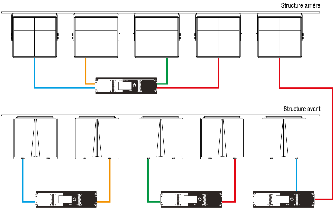
5 B218 et 5 M210 amplifiés par 4 NXAMP4X4MK2 sur deux structures séparées
